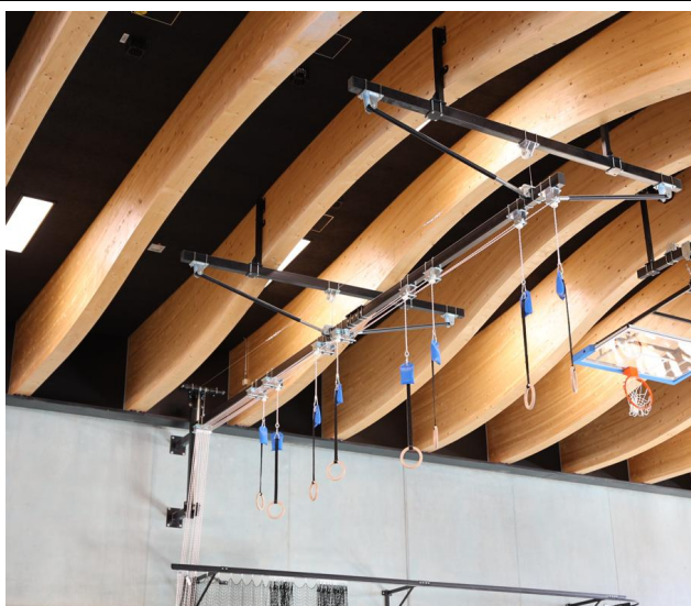
ASK-Anlage Teleskop-Abhängekonstruktion 81495 (4-Ringe) elektrisch hochziehbar (Beispielfoto für alle weiteren baugleichen Ausführungen 81475; 81480; 81485; 81490; 81500; 81501 )
